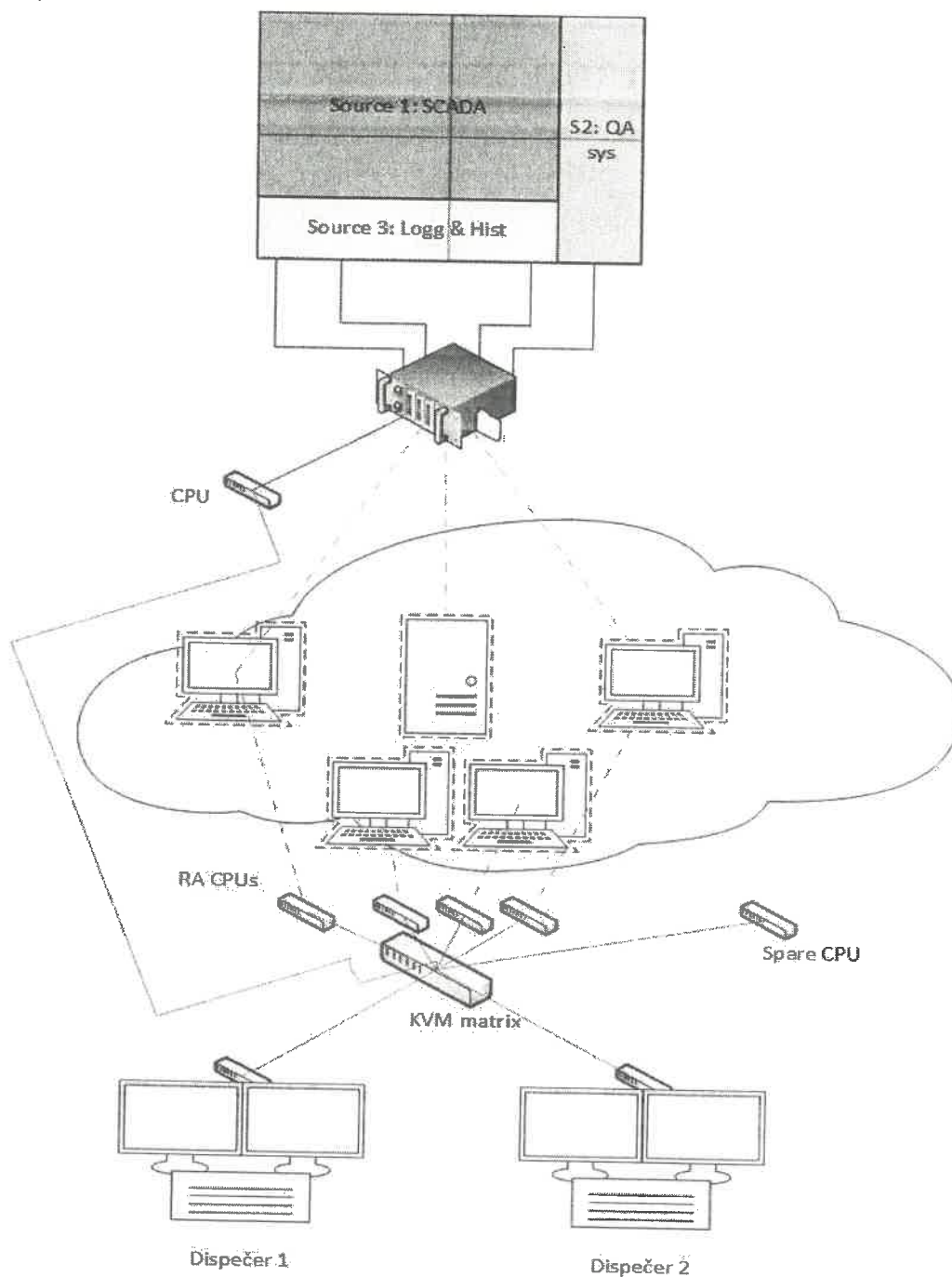
Slika 2. Osnovna koncepcija/Arhitektura sistema SCADA sistema (osnova za razradu tehničkog rješenja)
