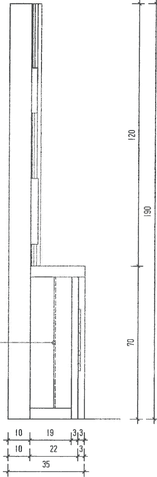
PRESJEK 1-1
